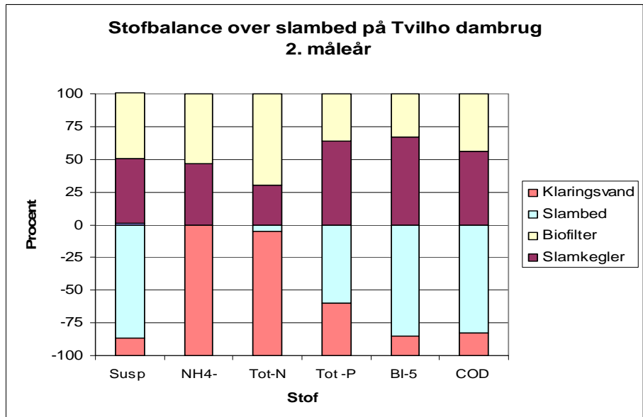
Figur 24 Stoffjernelse over slambassinerne på Tvilho Dambrug det andet måleår. Stoffinput til slambassinerne tilføres fra returskyllning af biofiltre og tømning af slamkegler i det samlede produktionsanlæg inkl. kummehus. Stoffindholdet i klaringsvandet er udtryk for den stofmængde, der tabes fra slambassinerne.
