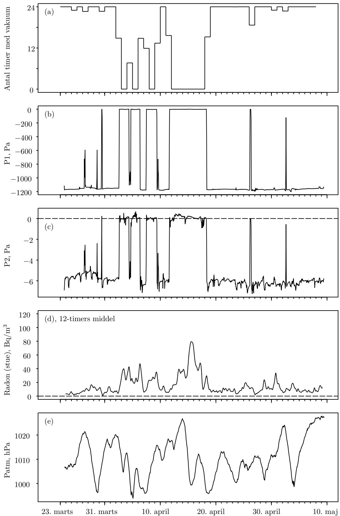
Figur A.16. Oversigt: (a) Drifttid for vakuumanlæg, (b) trykforskel mellem TB03 og hus, (c) do. mellem Gulv1 og hus, (d) radon i stuen, og (e) atmosfærisk tryk. Risø-R-1279(DA)
